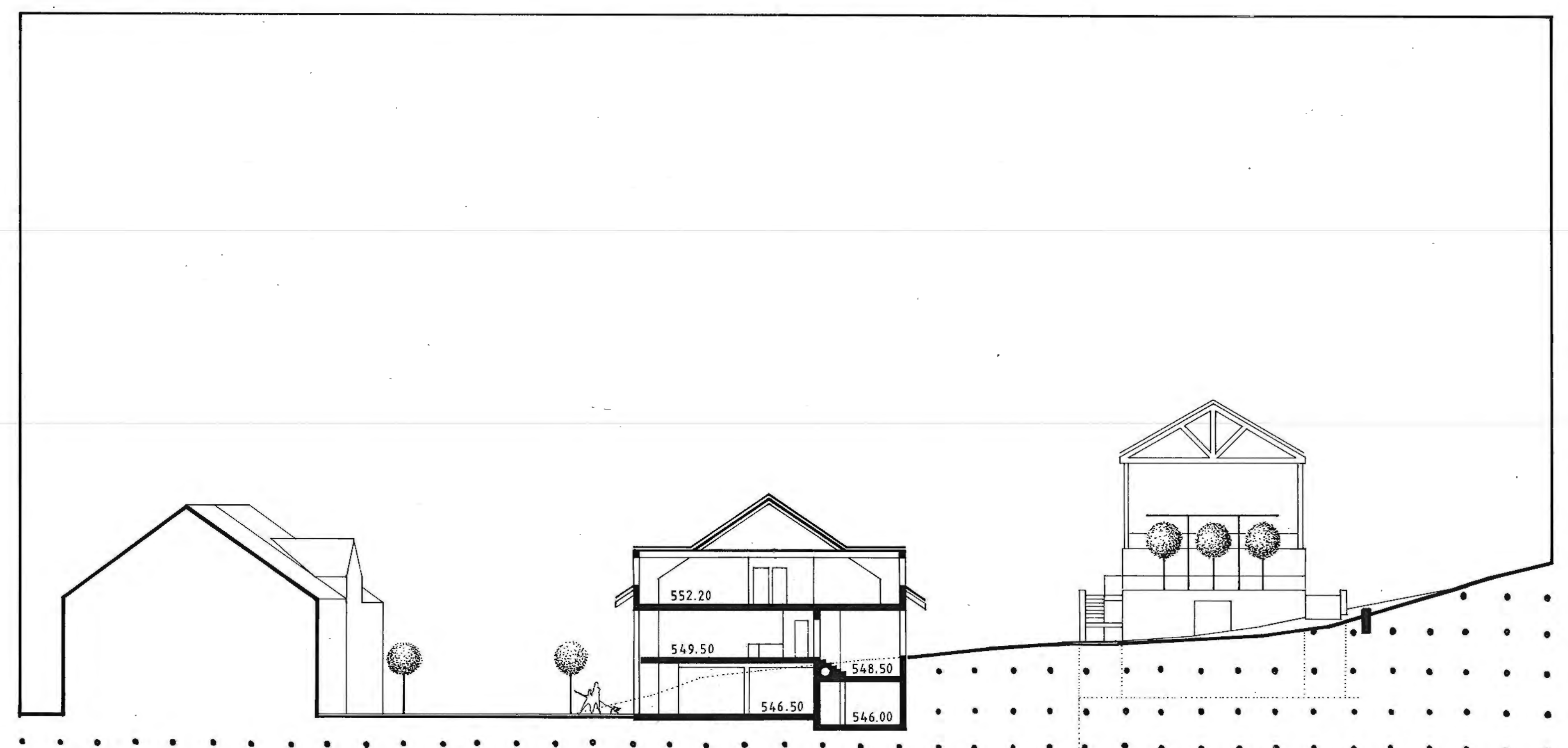
COUPE B-B
