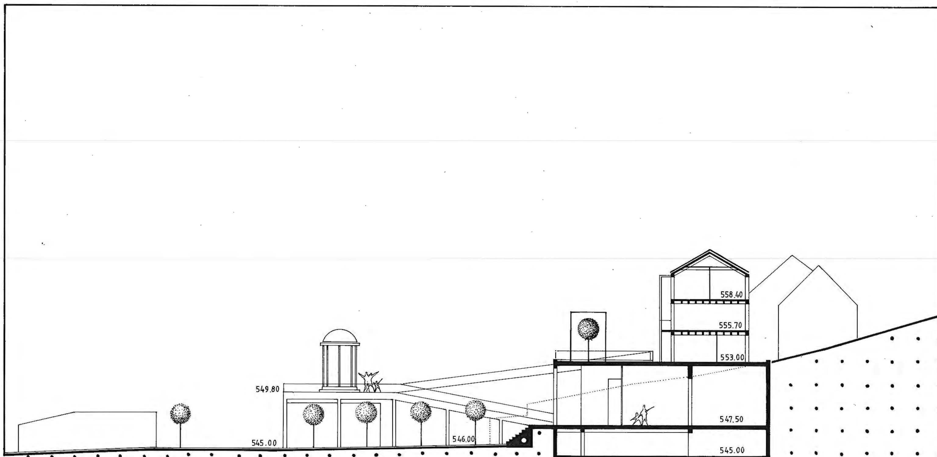
COUPE A-A
